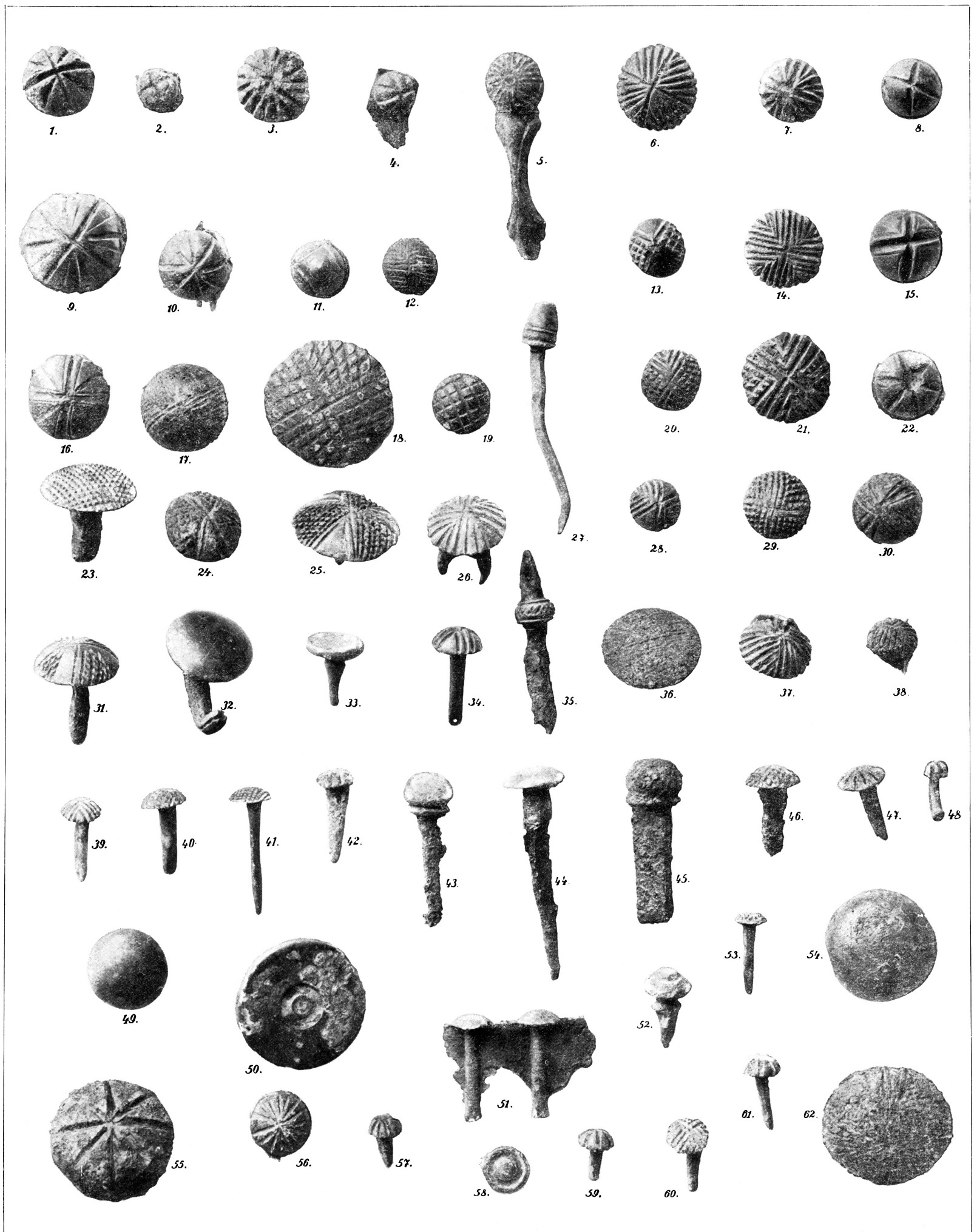
Ozdobné hlavičky bronzových hřebíků (vel. 1/1).
